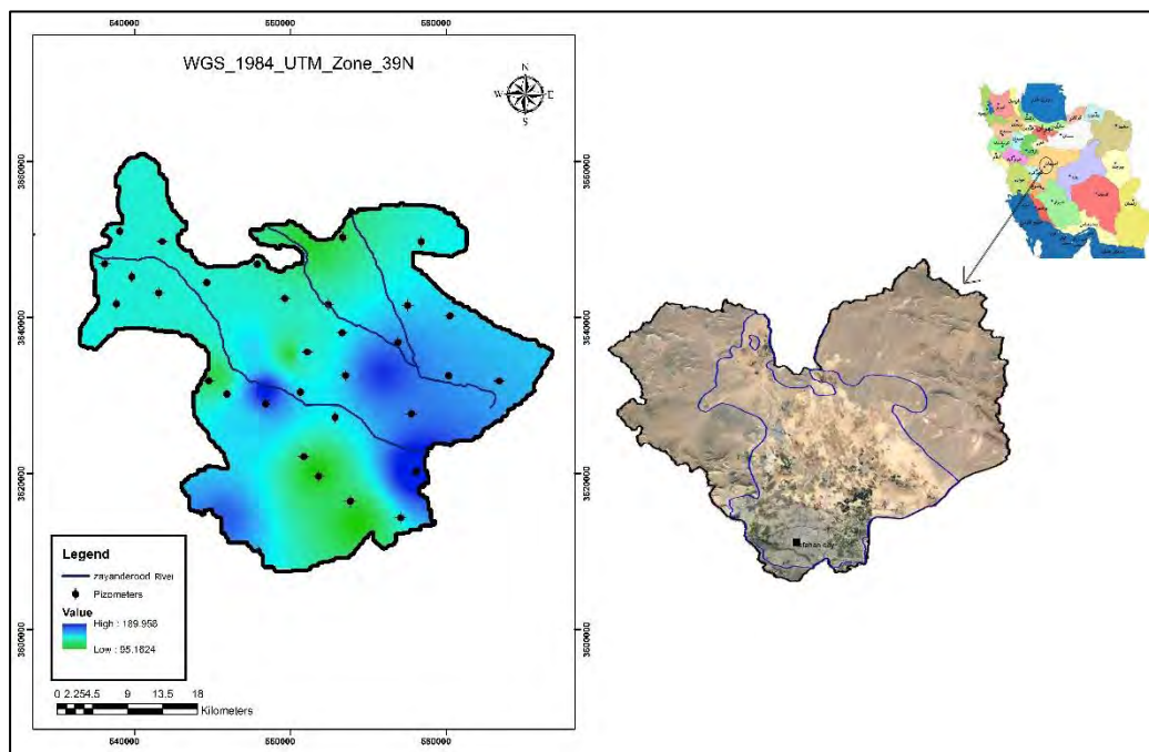
شکل ۱: موقعیت دشت و آبخوان و چاه‌های پیزومتری اصفهان-برخوار و نقشه‌ی هدایت هیدرولیکی
