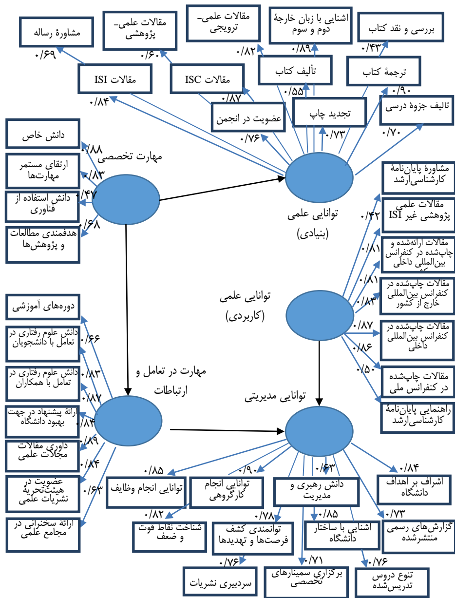
شکل ۲. مدل نهایی: مدل اجرایی پس از حذف شاخص‌های با بار عاملی کمتر از ۰/۴
