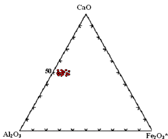
شکل ۶- نمایش موقعیت ترکیبی پرهنیت‌ها در دیاگرام \text{Al}_2\text{O}_3 - \text{CaO} - \text{Fe}_2\text{O}_3^* (Wheeler et al. , 2001).
