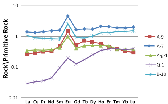
شکل ۱۰- نمودار به‌هنجار شده نمونه‌های دگرسان نسبت به سنگ اولیه
