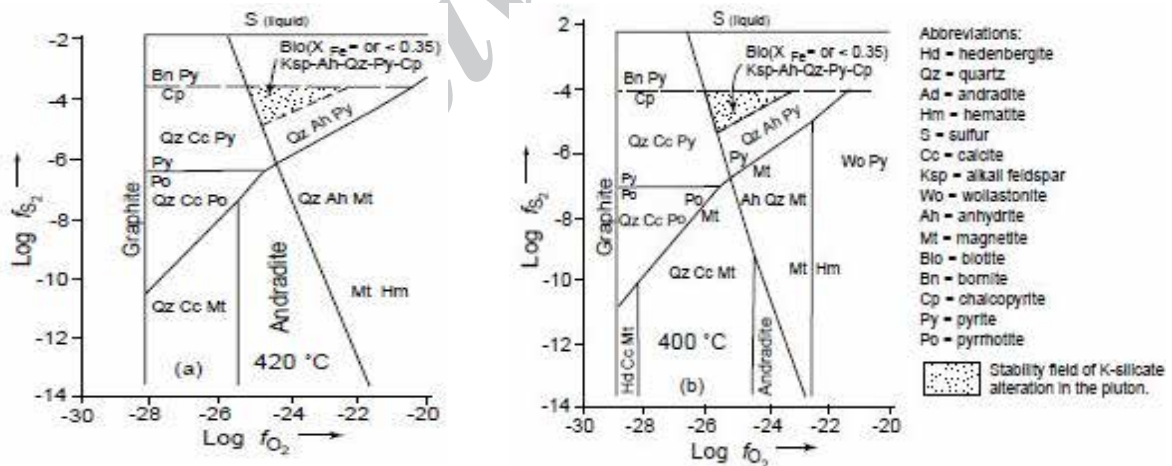
شکل ۱۷- نمودار دو متغیره \text{Log} f_{S_2} نسبت به \text{Log} f_{O_2} برای گستره پایداری آندرادیت در دماهای 400^\circ\text{C} و 420^\circ\text{C} و X_{CO_2} = 0.1 (Taylor and liou, 1978)
