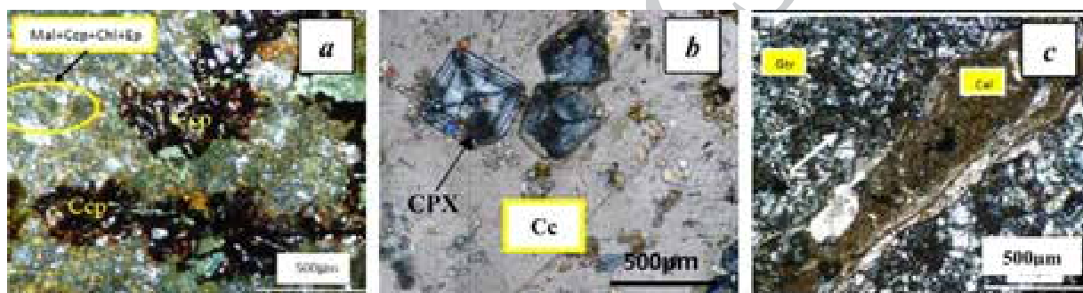
شکل ۶- تصاویر میکروسکوپی XPL از زون گارنت- پیروکسن اسکارن در منطقه خوت، (a) تبدیل کامل گارنت به کالکوپیریت، مالاکیت، اپیدوت و کلریت در زون گارنت- پیروکسن اسکارن‌های منطقه خوت در مرحله متاسوماتیسم پیش‌رونده، (b) ادخال‌های کلینوپیروکسن در گارنت‌های منطقه خوت و (c) کلسیت به‌صورت رگچه‌ای فضای بین گارنت‌های اینزوتروپ را پر نموده است.
