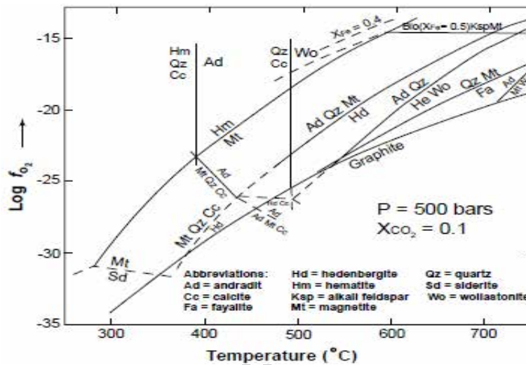
شکل ۱۶- روابط فازی T-log f_{O_2} در P = 500 bars و X_{CO_2} = 0.1 برای سامانه Ca-Fe-Si-C-O-H (Einaudi and Burt, 1982)
