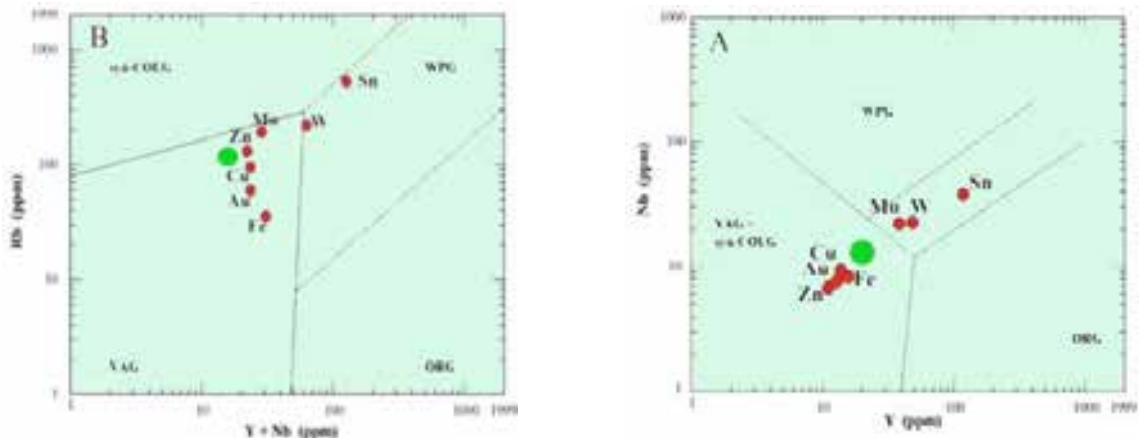
شکل ۱۰- نمودارهای تعیین‌کننده خاستگاه تکتونیکی گرانیتوئید خوت بر اساس عناصر کیمیا (Pearce et al., 1984). میانگین ترکیب نمونه‌های گرانیتوئید خوت. ●: میانگین ترکیب توده‌های نفوذی مرتبط با کانسارهای اسکارنی (Meinert, 1995)
