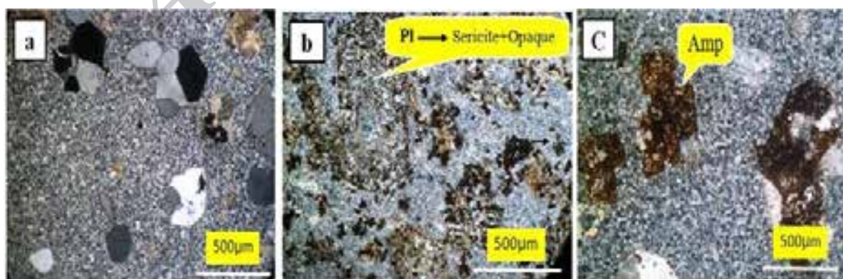
شکل ۴- تصاویر میکروسکوپی (XPL) از توده نفوذی پورفیری در منطقه خوت، (a) خوردگی خلیجی و گردشگی بلورهای کوارتز در گرانودیوریت‌های منطقه خوت، (b) جانشینی کامل پلاژیوکلازها با سریسیت و اپاک و (c) جانشینی کامل آمفیبول‌ها توسط اپاک در گرانیت‌های منطقه خوت
