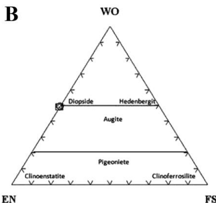
شکل ۸- A) موقعیت کلینوپیروکسن بر روی دیاگرام Q-J و تعیین گروه آن (Morimoto and Kitamura, 1983)، B) دیاگرام مثلثی Wo-En-Fs و تعیین نوع کلینوپیروکسن (Morimoto and Kitamura, 1983).
