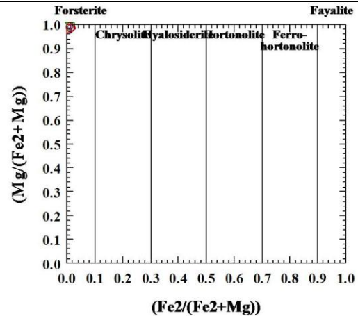
شکل ۹- نمودار تقسیم‌بندی الیون‌ها (Deer et al., 1972)
