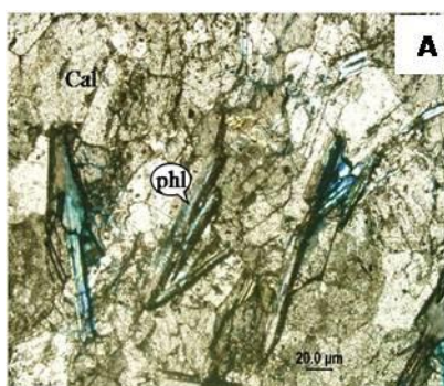
شکل ۵- A) تراکم ریزدانه‌های فلوگوپیت همراه با کلسیت در مرم‌های میکادار (XPL)، B) بلورهای کشیده مارگاریت در
