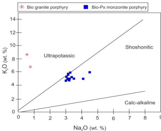
شکل ۷- موقعیت توده‌های نفوذی نیمه‌عمیق شمال شرقی نایبند در نمودار اکسید پتاسیم در مقابل اکسید سدیم (Chung et al., 1998)
