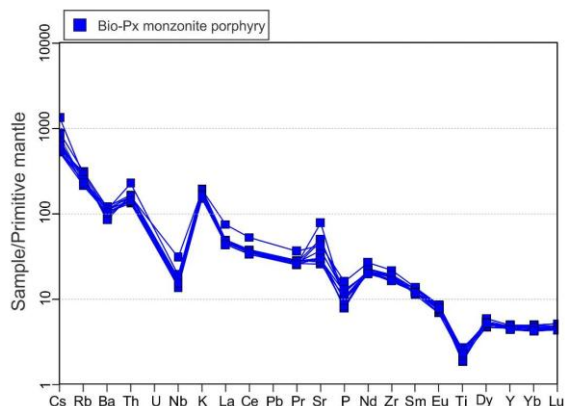
شکل ۱۱- نمودار نرمالیزه شده برخی عناصر فرعی و نادر خاکی توده مونزونیتی نسبت به گوشته اولیه (Sun and Mc Donough, 1989).
