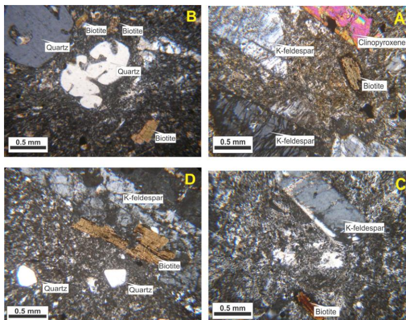
شکل ۴- تصاویری از مقاطع میکروسکوپی توده‌های نفوذی نیمه‌عمیق (ساب‌ولکان) منطقه بررسی شده در نور XPL، (A) واحد بیوتیت-پیروکسن موزونیت پورفیری، (B) واحد بیوتیت-کوارتز موزونیت پورفیری، (C) واحد بیوتیت-سینیت پورفیری، (D) واحد بیوتیت-گرانیت پورفیری
