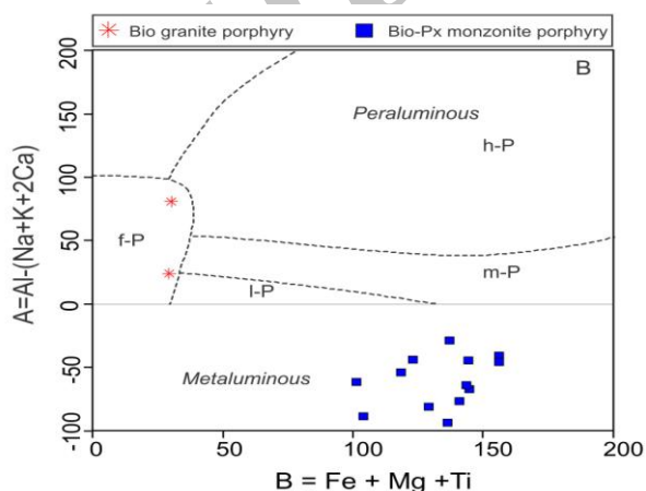
شکل ۶- A) موقعیت توده‌های نفوذی نیمه‌عمیق شمال شرقی نایبند در نمودار A/NK-A/CNK (Maniar and Piccoli, 1989). مرز جداکننده گرانیتوئیدهای نوع I و S در A/CNK=1.1 (Chappell and White 2001)؛ B) موقعیت توده‌های نفوذی نیمه‌عمیق شمال شرقی نایبند در نمودار چند کاتیونی تغییر یافته H-P، (Villaseca et al., 1998). H-P = گرانیتوئیدهای به شدت پرآلومینوس، M-P = گرانیتوئیدهای متوسط پرآلومینوس، L-P = گرانیتوئیدهای کم پرآلومینوس، F-P = گرانیتوئیدهای به شدت فلسیک
