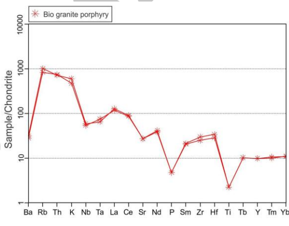
شکل ۱۲- نمودار نرمالیزه شده برخی فرعی و نادر خاکی توده گرانیتی نسبت به کندریت (Thompson, 1982)
