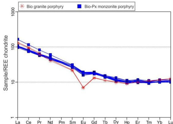
شکل ۱۰- نرمالیزه کردن عناصر نادر خاکی نسبت به کندریت در توده‌های نفوذی نیمه عمیق شمال شرقی نایبند (Boynton, 1985).
