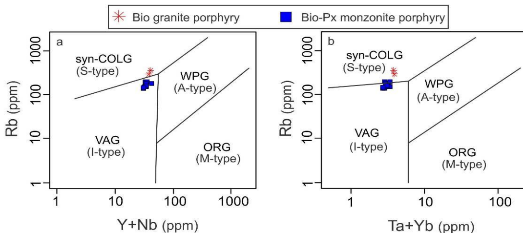
شکل ۹- موقعیت توده‌های نفوذی نیمه‌عمیق شمال شرقی نایبند در نمودار Pearce و همکاران (۱۹۸۴) تغییر یافته توسط Christiansen و Keith (۱۹۹۶). VAG = گرانیتوئیدهای قوس آتشفشانی، WPG = گرانیتوئیدهای درون صَفح‌های، ORG = گرانیتوئیدهای پشته میان اقیانوسی، syn-COLG = گرانیتوئیدهای همزمان با تصادم قاره‌ها.
