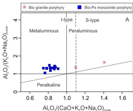
شکل ۶- A) موقعیت توده‌های نفوذی نیمه‌عمیق شمال شرقی نایبند در نمودار A/NK-A/CNK (Maniar and Piccoli, 1989). مرز جداکننده گرانیتوئیدهای نوع I و S در A/CNK=1.1 (Chappell and White 2001)؛ B) موقعیت توده‌های نفوذی نیمه‌عمیق شمال شرقی نایبند در نمودار چند کاتیونی تغییر یافته H-P، (Villaseca et al., 1998). H-P = گرانیتوئیدهای به شدت پرآلومینوس، M-P = گرانیتوئیدهای متوسط پرآلومینوس، L-P = گرانیتوئیدهای کم پرآلومینوس، F-P = گرانیتوئیدهای به شدت فلسیک
