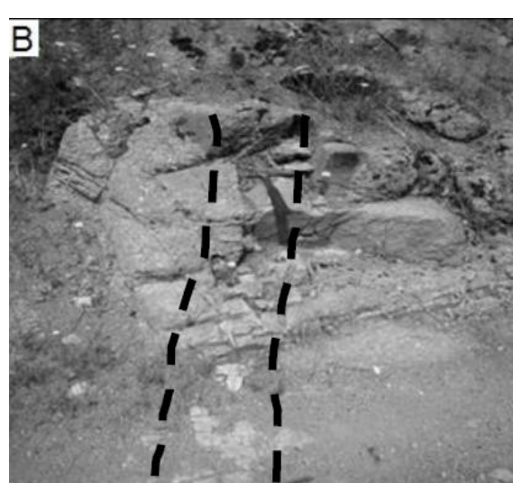
شکل ۳- A) واحد زمین‌شناسی (واحد EVP) رخنمون یافته در ۴۰ کیلومتری جاده زنجان-گیلوان، حوالی روستای بادامستان؛ B) رگه آپلیت، توده کوارتزموزنونیتی را قطع کرده است
