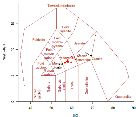
شکل ۶- A) طبقه‌بندی ژئوشیمیایی و نامگذاری سنگ‌های نفوذی با استفاده از مجموع آلكالی در برابر سیلیس (Middlemost, 1985)؛ B) نمودار K_2O در مقابل SiO_2 برای تمایز سری‌ها (Peccerillo and Taylor, 1976) (▲) مونزودیوریت، ■ مونزونیت، Δ کوارتز مونزونیت، ◆ مونزوگرانیت
