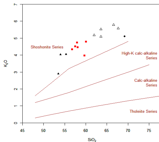
شکل ۶- A) طبقه‌بندی ژئوشیمیایی و نامگذاری سنگ‌های نفوذی با استفاده از مجموع آلكالی در برابر سیلیس (Middlemost, 1985)؛ B) نمودار K_2O در مقابل SiO_2 برای تمایز سری‌ها (Peccerillo and Taylor, 1976) (▲) مونزودیوریت، ■ مونزونیت، Δ کوارتز مونزونیت، ◆ مونزوگرانیت
