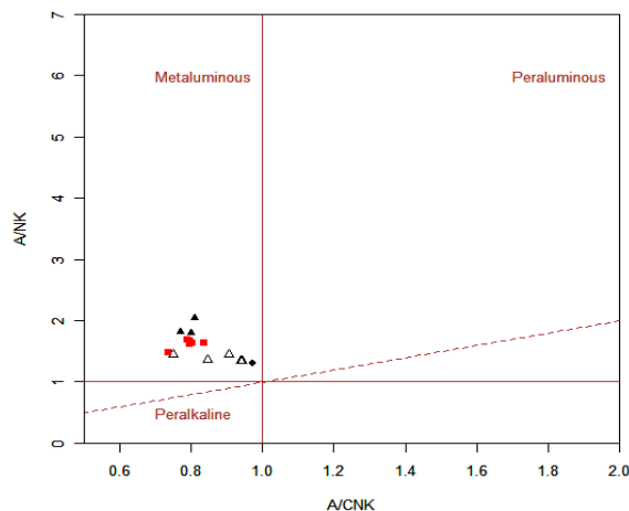
شکل ۷- نمودار A/NK در مقابل A/CNK برای تمایز ماگماهای پرآلومین، متآلومین و پرآلكالن (Maniar and Piccoli, 1989) و موقعیت نمونه‌های توده طارم علیا (▲) مونزودیوریت، ■ مونزونیت، Δ کوارتز مونزونیت، ◆ مونزوگرانیت
