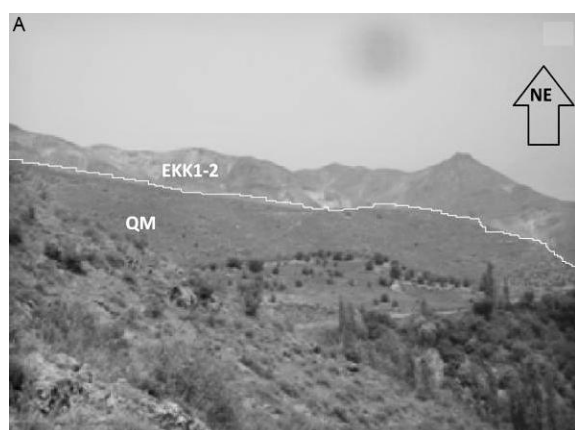
شکل ۲- A و B) واحدهای زمین‌شناسی (واحد EKK1-2 و توده نفوذی QM) رخنمون یافته در روستای زرده، در منتهی‌الیه جنوب‌شرقی توده
