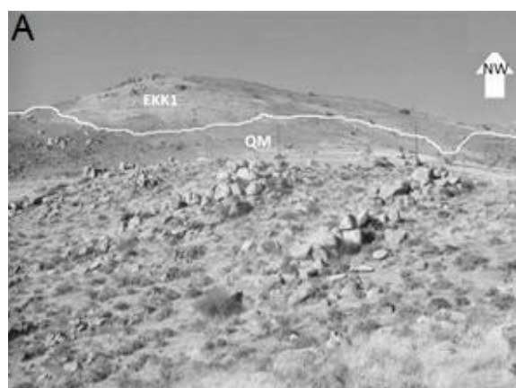
شکل ۱- A) واحدهای زمین‌شناسی (واحد EKK1 و توده نفوذی QM) رخنمون یافته در ۶۰ کیلومتری جاده زنجان-گیلوان، غرب روستای چفتان؛ B) در این شکل بخشی از رخنمون توده نفوذی (QM) مشاهده می‌شود که با سطح فرسایشی خشن‌تر و رنگ خاکی روشن از سنگ‌های میزبان (EKK1) قابل تشخیص است.
