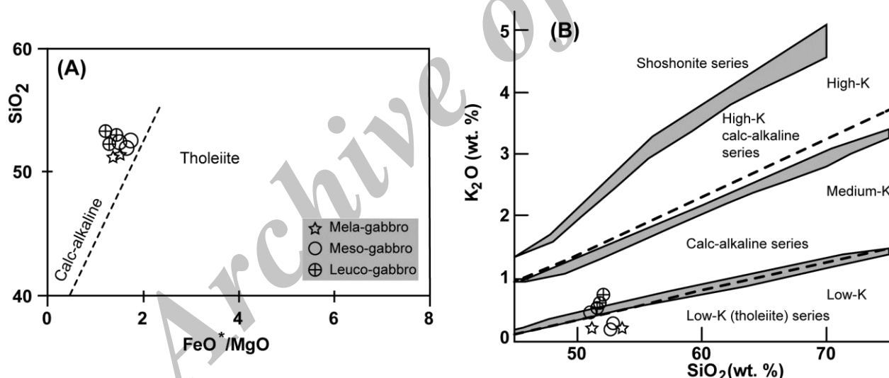
شکل ۶- نمونه‌های گابروهای خراجو (جنوب آذرشهر، آذربایجان شرقی) در نمودارهای توصیفی برای شناسایی سرشت ماگمایی در پهنه‌های فرورانشی: (A) نمودار اکسید عناصر اصلی \text{SiO}_2 (wt.%) در \text{FeO}^*/\text{MgO} (Miyashiro, 1974). نمونه‌ها در محدوده کالک‌آلکان جای دارند؛ (B) نمودار \text{K}_2\text{O} در برابر \text{SiO}_2 برای شناسایی سری ماگمایی در پهنه‌های فرورانشی (Rickwood, 1989). نمونه‌ها سرشت توله‌ایتی با پتاسیم کم تا کالک‌آلکان با پتاسیم متوسط نشان می‌دهند.
