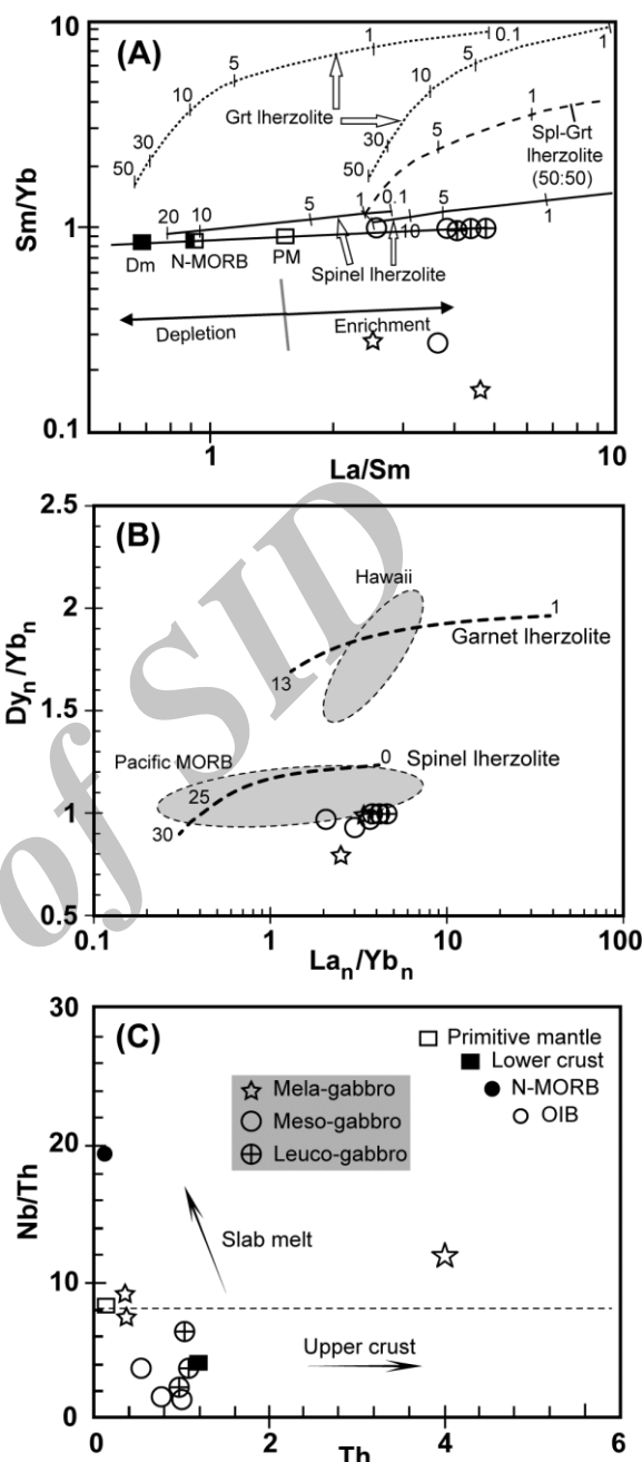
شکل ۸- نمودارهای عناصر ناسازگار نامتحرک و نسبت‌های آنها برای نمونه‌های گابرویی خراجو (جنوب آذرشهر، آذربایجان شرقی): (A) Sm/Yb در برابر La/Sm (Aldanmaz et al., 2000). MORB تهی‌شده (DM؛ McKenzie and O'Nions, 1991)، گوشته اولیه و MORB عادی (به‌ترتیب PM و N-MORB؛ Sun, 1989) (B) Dy n /Yb n در برابر La n /Yb n (and McDonough, 1989)؛ (C) Nb/Th (Rogers, 2015) برای شناسایی سنگ مادر اولیه؛ در برابر Th (به ppm). مقدار N-MORB و OIB و Primitive mantle از Sun and McDonough (1989) است.
