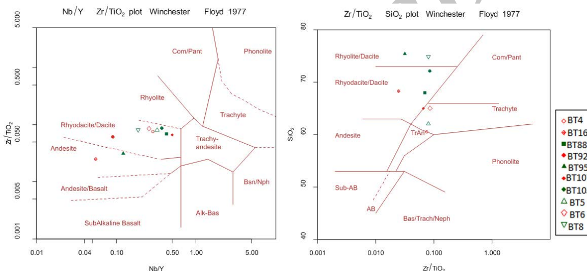
شکل ۸- رده‌بندی توف‌های منطقه حصاربن (جنوب‌باختری فیروزکوه) در نمودارهای پیشنهادی Winchester و Floyd (۱۹۷۷)
