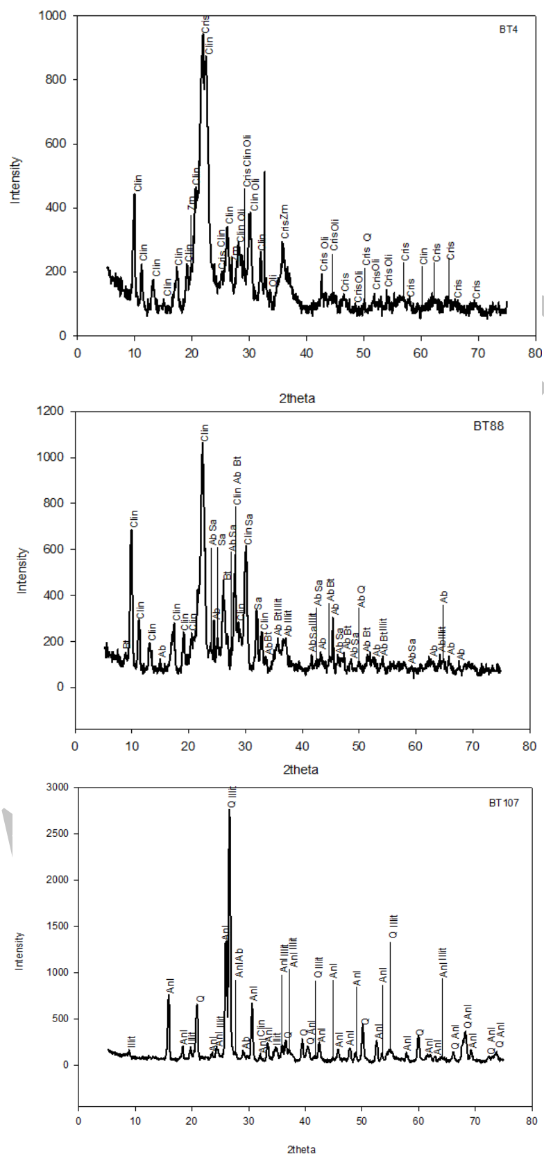
شکل ۷- پراش پرتوی ایکس نمونه‌های BT4، BT88، BT107 (توف‌های منطقه حصاربن، جنوب‌باختری فیروزکوه): Cris: کریستوبالیت؛ Clin: کلینوپتیلولیت؛ Oli: الیگوکلاز؛ Zm: زیرکن؛ Q: کوارتز؛ Bt: بیوتیت؛ Sa: سانیدین؛ Ab: آلبیت؛ Anl: آنالسیم؛ Illit: ایلیت)
