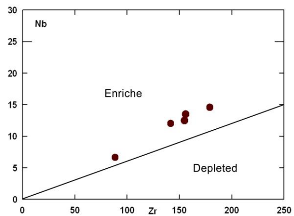
شکل ۲۶- نمونه‌های آتشفشانی جیرنده (شمال‌باختری قزوین) در نمودارهای غنی‌شدگی و با تهی‌شدگی ناحیه خاستگاه (Abu-Hamattah, 2005)
