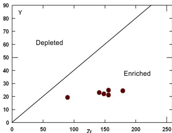
شکل ۲۶- نمونه‌های آتشفشانی جیرنده (شمال‌باختری قزوین) در نمودارهای غنی‌شدگی و با تهی‌شدگی ناحیه خاستگاه (Abu-Hamattah, 2005)
