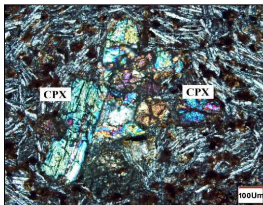
شکل ۶- تصویر میکروسکوپی (XPL) از بافت گلوپورفیری پدیدآمده از انباشتگی بلورهای پروکسن در زمینه‌ای میکروولیتی ساخته شده از پلاژیوکلازها (بازالت جیرنده، شمال باختری قزوین)
