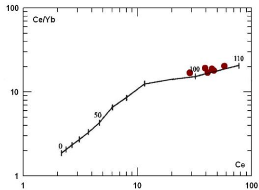
شکل ۲۵- نمونه‌های آتشفشانی جیرنده (شمال‌باختری قزوین) در نمودار Ce در برابر Ce/Yb (Ellam and Cox, 1991)
