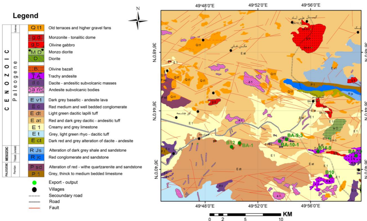
شکل ۱- نقشه زمین‌شناسی منطقه جیرنده در شمال‌خاوری قزوین (رسم دوباره‌ای از نقشه ۱:۱۰۰۰۰۰ جیرنده (Ghalamghash, 2002))
