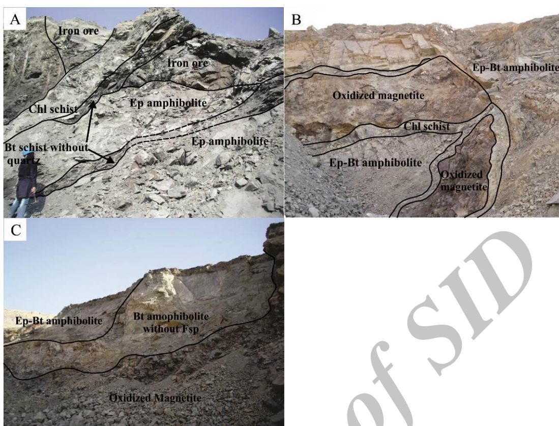
شکل ۳- نمای صحرایی آمفیبولیت‌های معدن سنگ آهن گل‌گهر (کرمان): (A) نمایی از اپیدوت آمفیبولیت در کنار سنگ آهن. در کناره سنگ آهن و نیز درون اپیدوت آمفیبولیت، نوار باریکی از بیوتیت شیبست بی کوارتز دیده می‌شود؛ (B) نمایی از نفوذ سنگ آهن درون اپیدوت- بیوتیت آمفیبولیت که در پیرامون آن هاله سبز رنگ کلریت شیبست دیده می‌شود (دیواره شمالی پله ۱۱ باختری، دید رو به شمال؛ C) نمایی از بیوتیت آمفیبولیت بی فلدسپار و دگرسان‌شده و اپیدوت- بیوتیت آمفیبولیت در کنار سنگ آهن اکسیدشده (دیواره شمالی پله ۱۱ باختری، دید رو به شمال‌باختری) (Chl: کلریت؛ Amp: آمفیبول؛ Bt: بیوتیت؛ Ep: اپیدوت؛ نام اختصاری کانی‌ها از Whitney و Evans (۲۰۱۰) برگرفته شده است)
