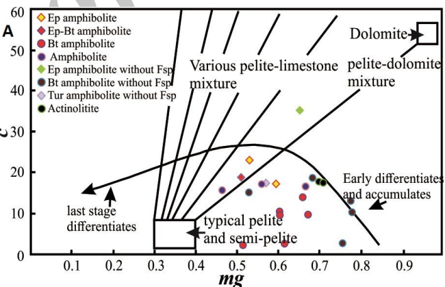
شکل ۷- آمفیبولیت‌های معدن سنگ آهن گل‌گهر سیرجان در: (A) نمودار mg نیگلی در برابر c ، خط روند جدایش بلوری ماگمایی دولریت‌های کارو و دیگر خط‌ها مخلوط‌های آهک-دولومیت را که با مقادیر متغیر پلیت و سمی پلیت آمیخته شده‌اند را نشان می‌دهد (Leake, 1964)؛ (B) نمودار c نیگلی در برابر al-alk (Evans and Leake, 1960)
