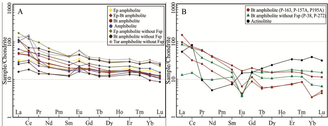
شکل ۱۵- ترکیب آمفیبولیت‌های معدن گل‌گهر سیرجان در: (A) نمودار عنصرهای خاکی نادر بهنجارشده به ترکیب کندریت (Boynton, 1984) (برای برخی آمفیبولیت‌های کلریت‌دار منطقه) (B) نمودار عنصرهای خاکی نادر بهنجارشده به ترکیب کندریت (Boynton, 1984)
