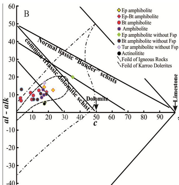
شکل ۷- آمفیبولیت‌های معدن سنگ آهن گل‌گهر سیرجان در: (A) نمودار mg نیگلی در برابر c ، خط روند جدایش بلوری ماگمایی دولریت‌های کارو و دیگر خط‌ها مخلوط‌های آهک-دولومیت را که با مقادیر متغیر پلیت و سمی پلیت آمیخته شده‌اند را نشان می‌دهد (Leake, 1964)؛ (B) نمودار c نیگلی در برابر al-alk (Evans and Leake, 1960)
