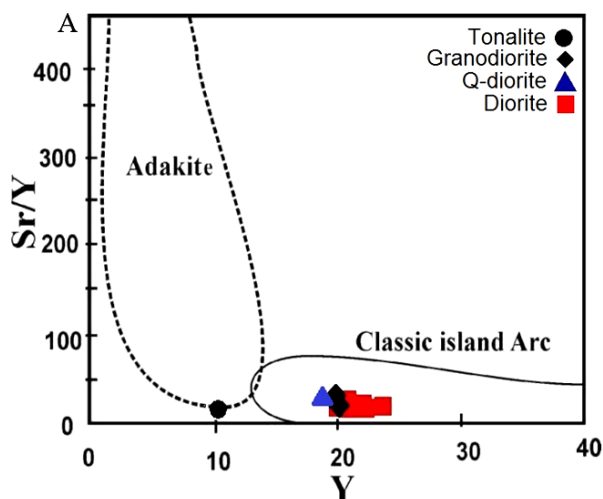
شکل ۱۳- سنگ‌های گرانیتوئیدی محدوده حنار در: (A) نمودار Y در برابر Sr/Y (Defant and Drummond, 1990); (B) نمودار Yb_N در برابر (La/Yb)_N (Martin, 1994)
