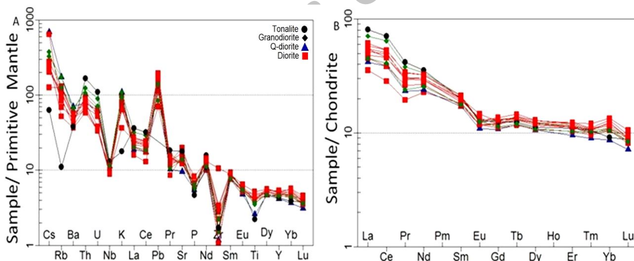
شکل ۸- نمونه‌های گرانیتوئیدی منطقه حنار (جنوب بیرجند) در: (A) نمودار الگوی عنصرهای کمیاب بهنجار شده به ترکیب گوشته اولیه (Sun and McDonough, 1989)؛ (B) الگوی عنصرهای خاکی نادر بهنجار شده به ترکیب کندریت (Boynton, 1984)
