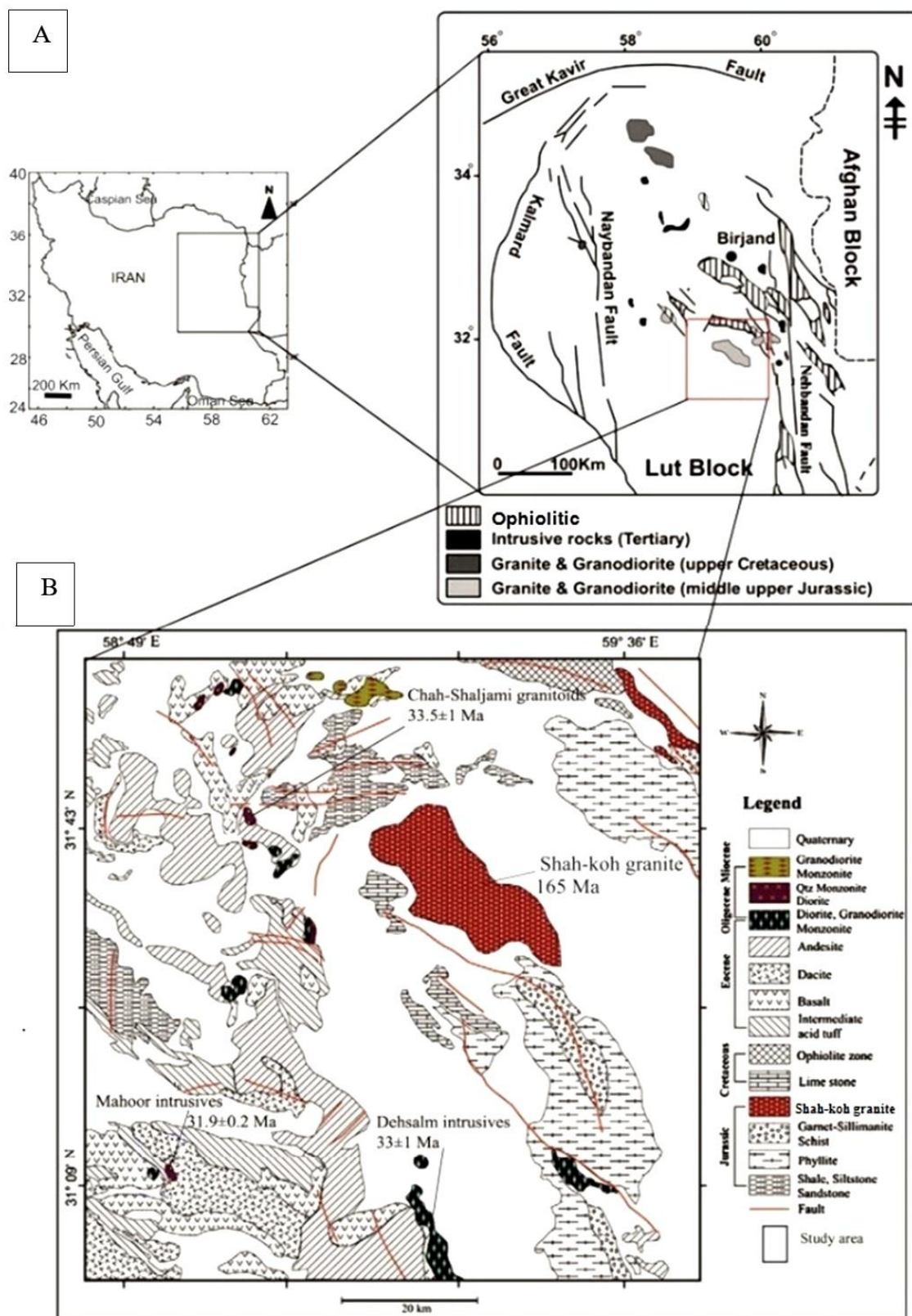
شکل ۱- A) موقعیت ساختاری بخش شمالی بلوک لوت (برگرفته از: Berberian و King (۱۹۸۱)، با اندکی تغییر); B) جایگاه رخنمون توده نفوذی محدوده حنار در بخش شمالی پهنه آتشفشانی-نفوذی بلوک لوت (برگرفته از: Arjmandzadeh و همکاران (۲۰۱۱b)، با تغییرات)
