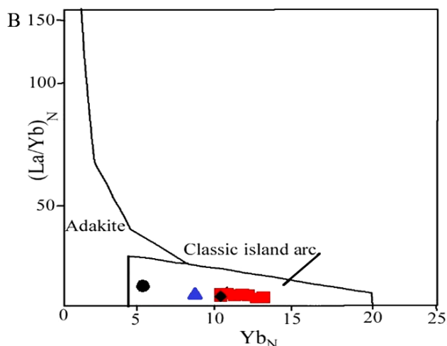
شکل ۱۳- سنگ‌های گرانیتوئیدی محدوده حنار در: (A) نمودار Y در برابر Sr/Y (Defant and Drummond, 1990); (B) نمودار Yb_N در برابر (La/Yb)_N (Martin, 1994)
