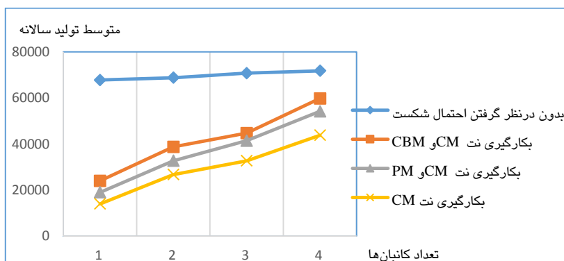
شکل ۴- تاثیر تعداد کانبان‌ها و سیاست‌های نگهداری و تعمیرات بر میزان تولید
