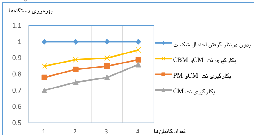
شکل ۶- تاثیر تعداد کانبان‌ها و سیاست‌های نگهداری و تعمیرات بر بهره‌وری دستگاه‌ها
