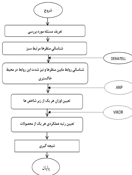
شکل ۱- مراحل تحقیق
