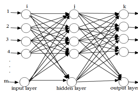
نگاره‌ی (۱): شبکه پرسپترون چند لایه‌ای
