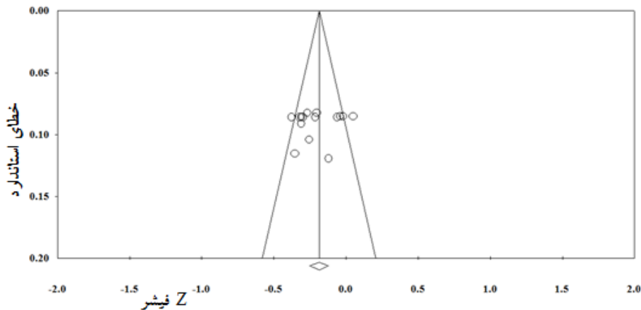
تصویر ۲: نمودار کیفی تورش انتشار بر اساس اثرهای تصادفی در پژوهش‌های انجام‌شده در حوزه رابطه‌ی انگیزه‌های اجتنابی فداکاری و کیفیت زناشویی
