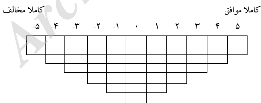
شکل (۱) نمودار کیو و نحوه مرتب سازی عبارات
