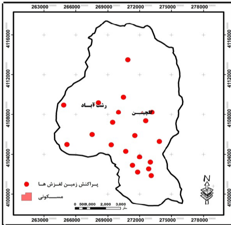
شکل (۲) نقشه پراکنده‌گی زمین لغزش محدوده
