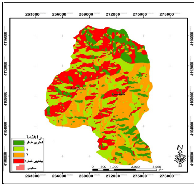
شکل (۹) نقشه جهت شیب حوضه
