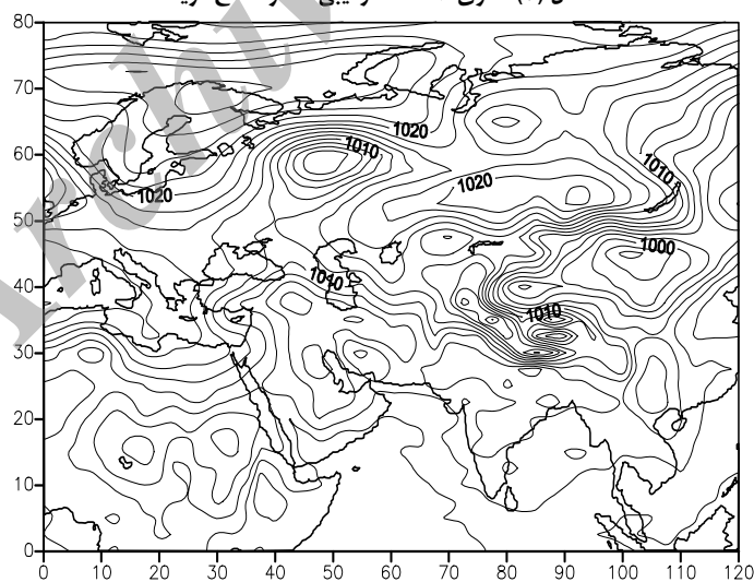
شکل (۸) روز نماینده الگوی ۳ فشار سطح دریا
