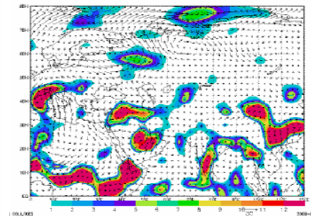
a همگرایی شار رطوبت در ساعت ۰۰:۰۰
