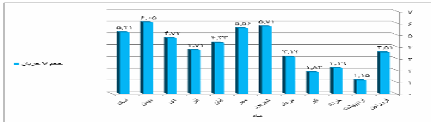
شکل (۳) نمودار درصد حجم آبدهی ماهیانه حوضه شمرود (ماخذ: نویسندگان)
