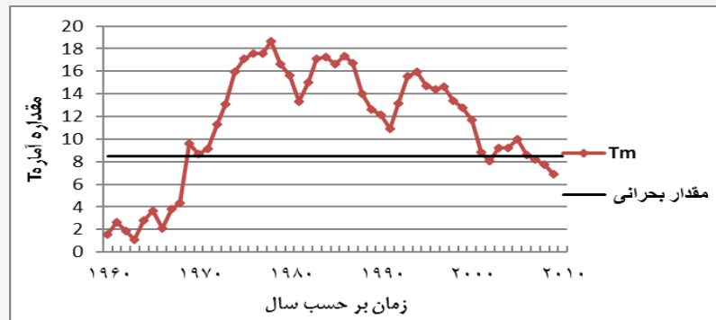
شکل (۴) تغییرات آماره دمای کمینه فصل تابستان ایستگاه رشت از روش آزمون همگنی نرمال استاندارد مطلق
