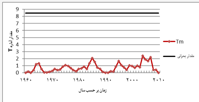
شکل (۵) تغییرات آماره دمای بیشینه سالانه ایستگاه رشت از روش آزمون همگنی نرمال استاندارد نسبی
