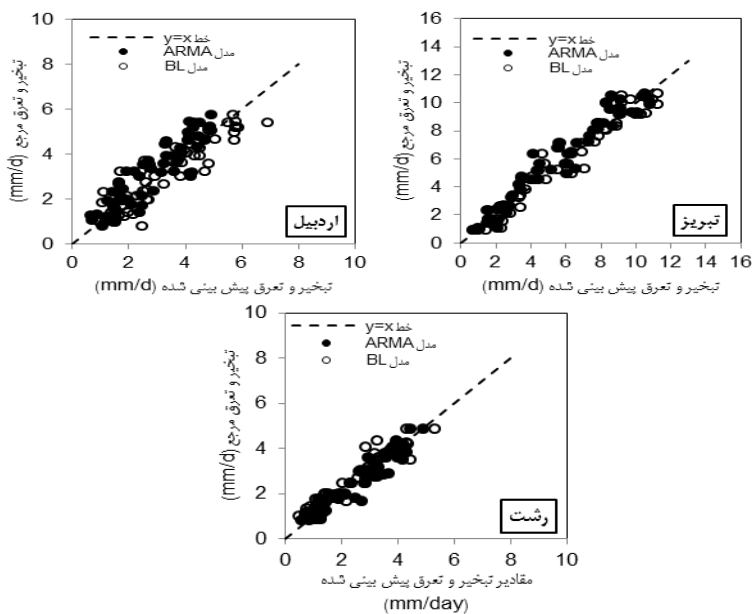
شکل (۲) مقایسه مقادیر پیش‌بینی شده ET_0 توسط مدل‌های خطی و غیرخطی با مبنای قرار دادن مقادیر تبخیر و تعرق مرجع در مرحله صحت‌سنجی (خط چین: خط y=x )
