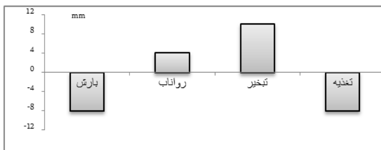
شکل ۵- اختلاف میانگین سالانه بارش، رواناب، تاخیر و تغذیه برای دوره 2013-2022 نسبت به دوره مبنا در حوضه آبریز تسوج با استفاده از مدل HADCM3 و سناریوی A2
