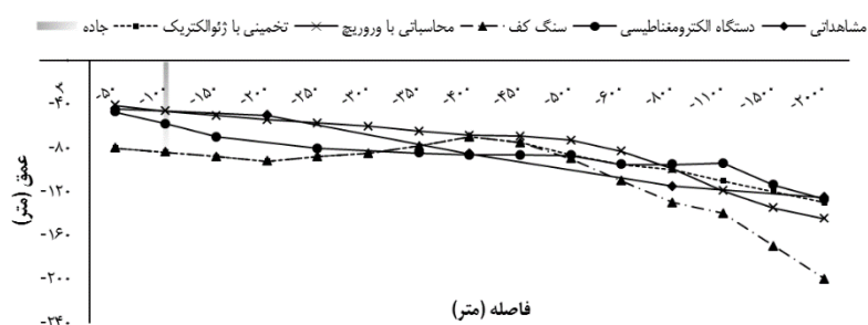
شکل ۶. مقایسه نتایج مطالعات مختلف تعیین حد تداخل آب شور و شیرین در مقطع دوم نوره
