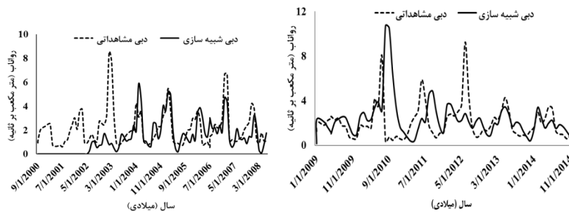
شکل (۳) شبیه‌سازی دبی حوضه یامچی با مدل IHACRES: الف) دوره واسنجی (ب) دوره اعتبارسنجی
