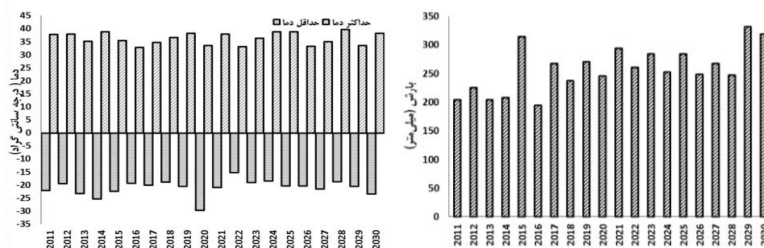
شکل (۲) نتایج پیش‌بینی مدل Lars با سناریو A1B: الف) بارندگی، ب) درجه حرارت حداقل و حداکثر
