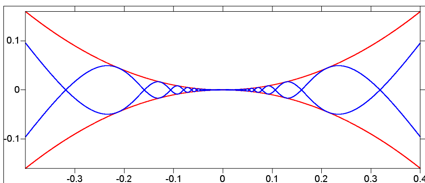
شکل (۳) ساختار کلاسیک فراکتال دو بعدی
