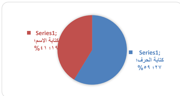
الرسم البياني - الرقم ٢: النسبة المئوية للكتابة الصحيحة للمفردات
