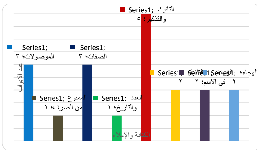
الرسم البياني - الرقم ٣: إملاء الأسماء
