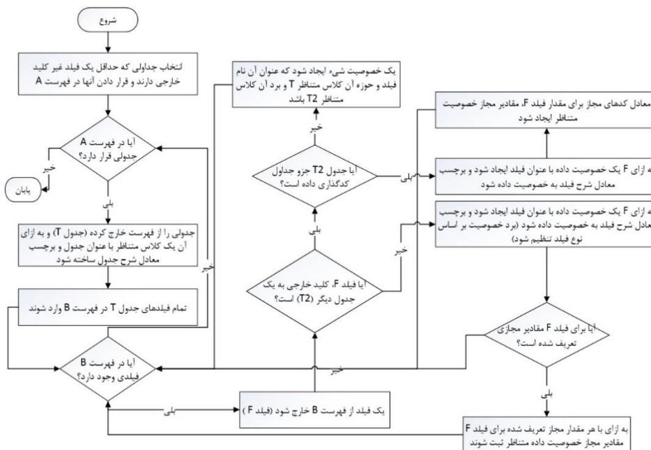
شکل ۳. نمودار گردش اعمال قوانین پایه، محدودیت و نوع داده
