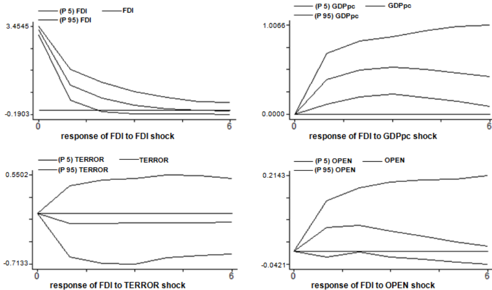
نمودار (۵): توابع عکس‌العمل آنی برای سرمایه‌گذاری مستقیم خارجی ورودی
