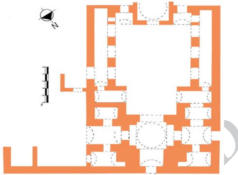
پلان شماره ۳: آتشکده رُهنی (Vanden Berghe, 1961)
