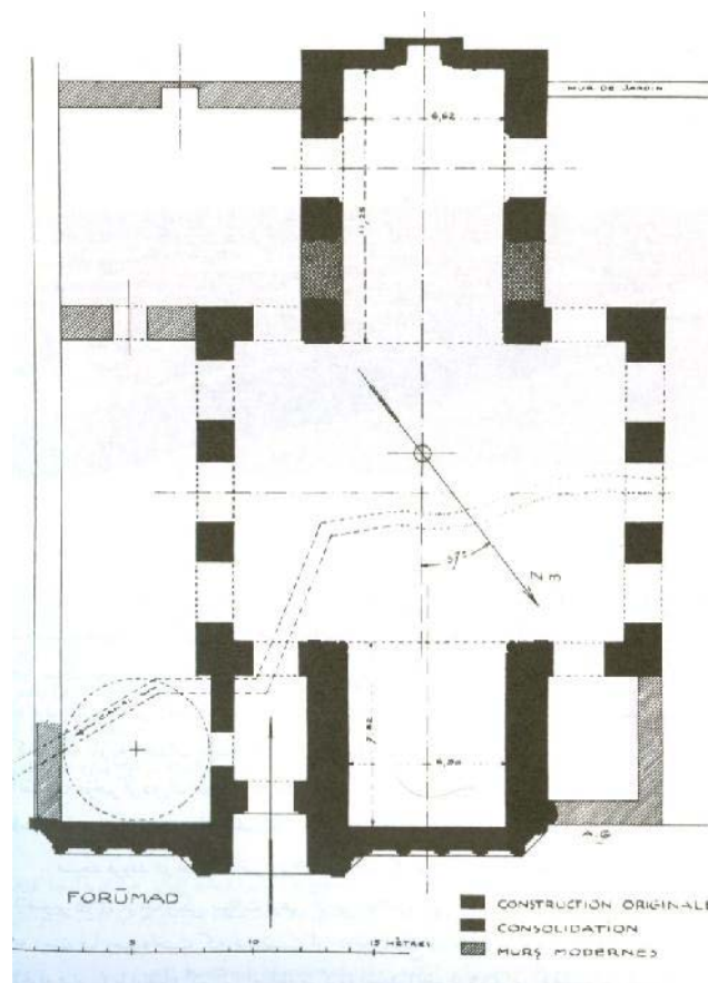
ش ۱، نقشه مسجد فرومد که به آندره گذار تهیه شده است (گذار، ۱۳۷۱، ج ۲: ۲۵۸).
