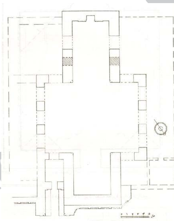
ش ۴، نقشه مسجد جامع فریومد ترسیم ویلبر (ویلبر، ۱۳۶۵: ۳۹ شماره فهرست ۶۱).
