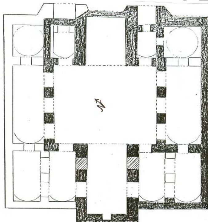
نقشه شماره ۷ مسجد جامع نقشه بازسازی شده براساس اطلاعات موجود
