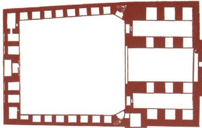
ش ۶، نقشه مسجد جامع قاین (لباف خانیکی، ۱۳۸۵: ۲۲).
