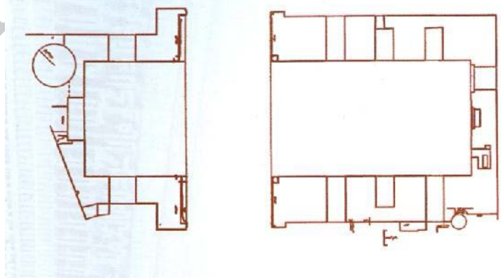
ش ۲، نقشه مسجد جامع ملک زوزن (لباف خانیکی، ۱۳۸۵: ۳۵).
