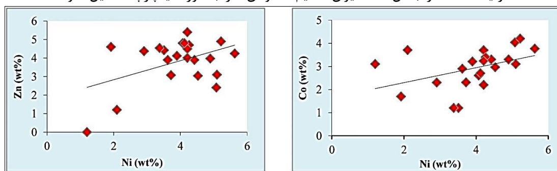
نمودار ۲- توزیع همبسته نیکل - کبالت (Ni-Co) و نیکل - روی (Ni-Zn) در نمونه‌های مورد مطالعه
