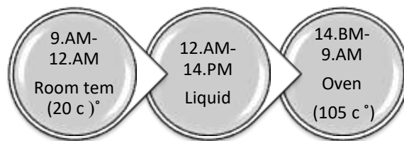
تصویر ۴. نمودار چرخه‌های آزمون شکستگی نمکی (مأخذ: نگارندگان)
