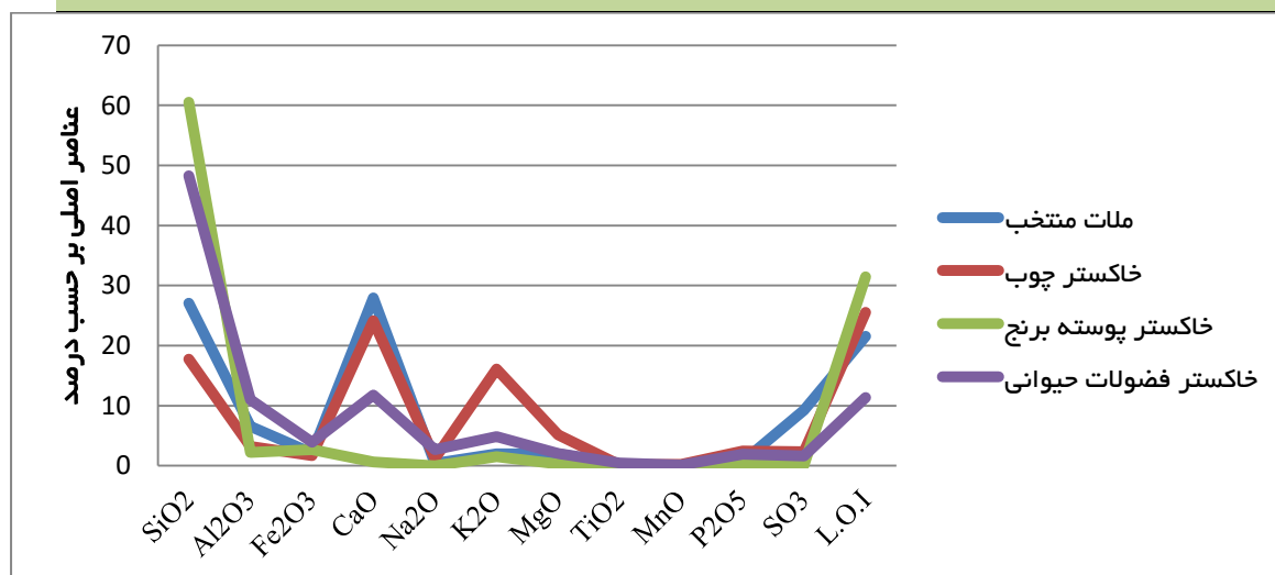
تصویر ۱۰. نمودار خطی مقایسه نتایج آنالیز شیمیایی پوزولان‌ها و نمونه ملاط متنخب بر اساس درصد وزنی اکسیدهای اصلی با استفاده از (XRF) (مأخذ: نگارندگان)
