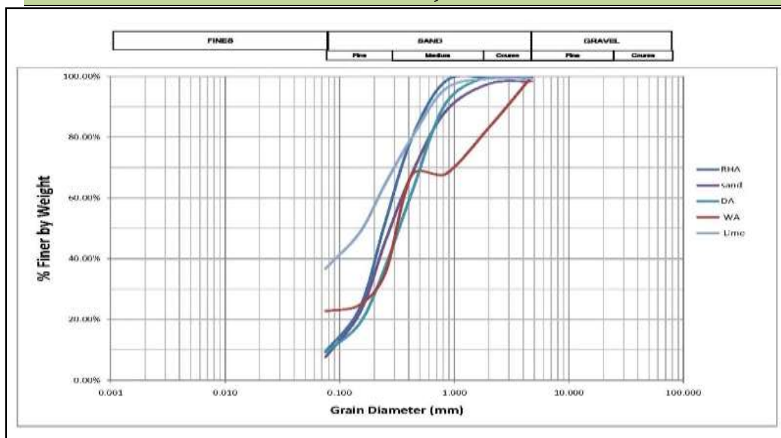
تصویر ۵. نمودار دانه‌بندی مصالح به کاررفته در نمونه‌های ملاط (مأخذ: نگارندگان)
