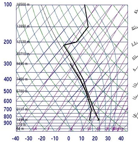
SkewT
