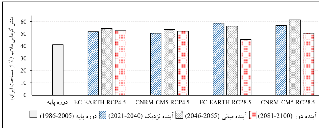
شکل ۷- اثر تغییر اقلیم بر تغییر مساحت پهنه‌های شامل تنش گرمایی ملایم ایران در فصل تابستان (واحد: % از مساحت ایران)
