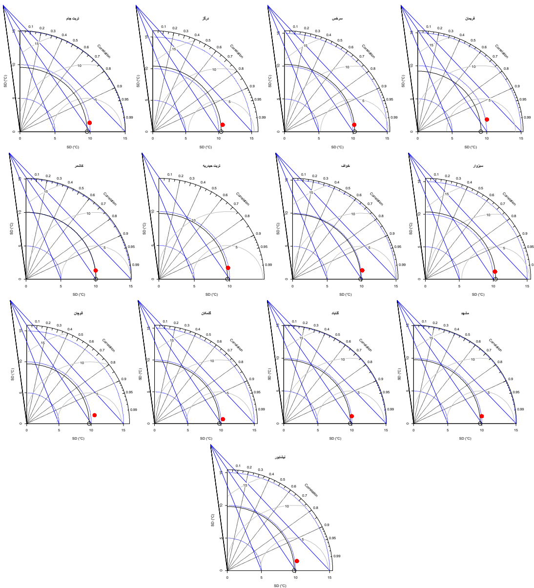
شکل ۳- مقایسه دمای میانگین ماهانه دمای بیشینه روزانه نقطه‌ای (ایستگاه‌های همدیدی خراسان رضوی) با شبکه‌ای CRU
