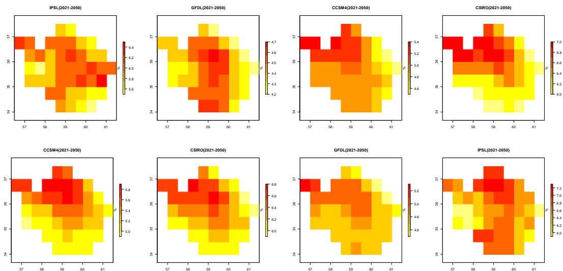
شکل ۱۰. درصد افزایش تبخیر-تعرق مرجع سالانه دوره ۲۰۲۱-۲۰۵۰ نسبت به دوره‌ی ۱۹۶۱-۲۰۰۵ تحت سناریوی RCP4.5 (بالا) و RCP8.5 (پایین)
