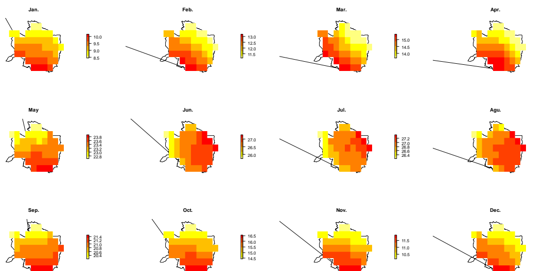
شکل ۴- داده‌های شبکه‌بندی شده‌ی تابش خورشیدی ماهانه برحسب مگاژول بر مترمربع بر روز (WorldClim, 2017)
