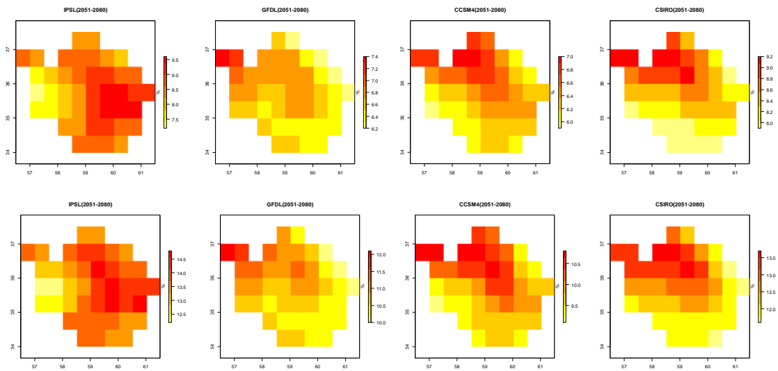
شکل ۱۱. درصد افزایش تبخیر-تعرق مرجع سالانه دوره ۲۰۵۱-۲۰۸۰ نسبت به دوره ۲۰۰۵-۹۶۱ تحت سناریوی RCP4.5 (بالا) و RCP8.5 (پایین)
