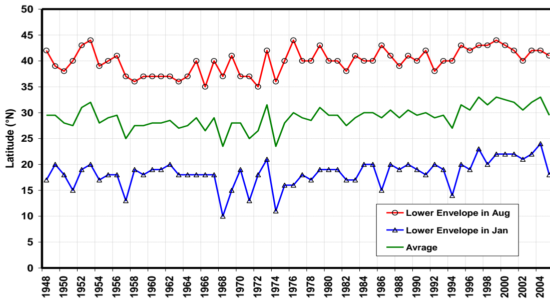
شکل ۸- تغییرات خط هم ارتفاع ۵۸۴ دکامتر در سطح ۵۰۰ هکتوپاسکال در طول جغرافیایی ۵۳ درجه شرقی طی ماه‌های ژانویه و آگوست در دوره ۱۹۴۸-۲۰۰۵ انتخاب شده برای ایران بعنوان پوش پایین جریانات غربی.
