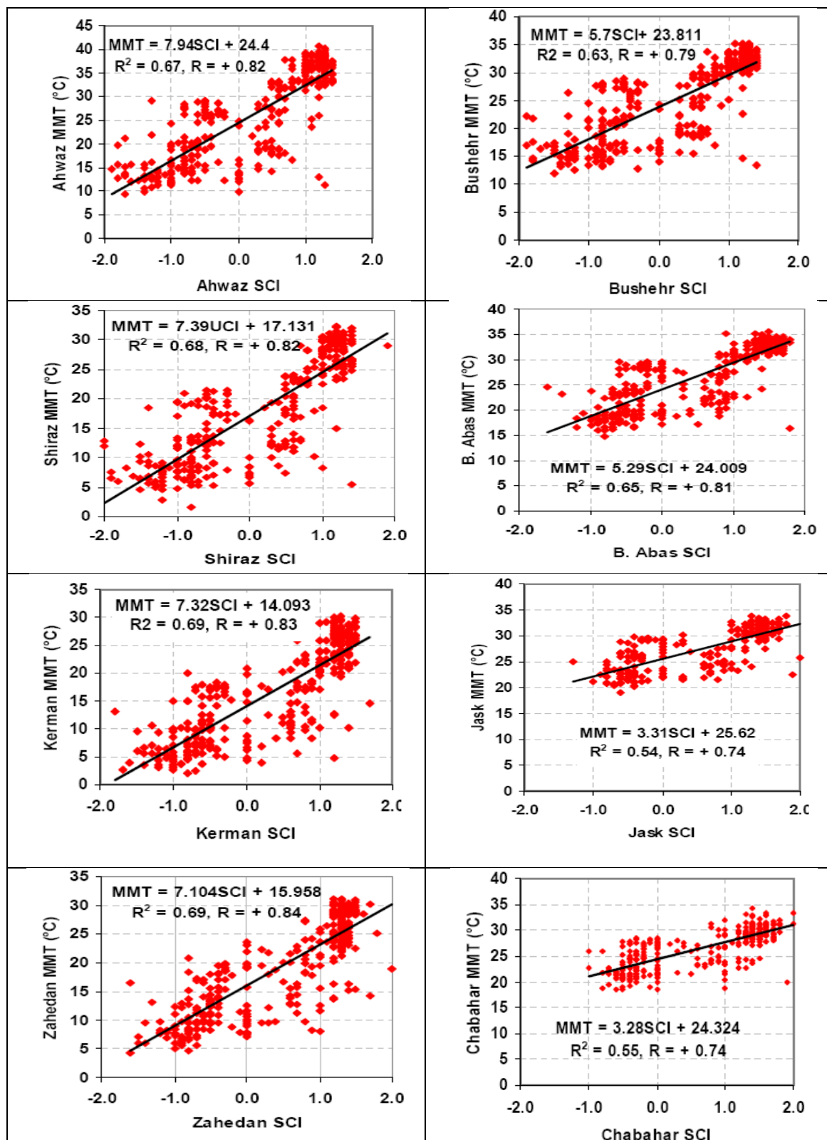
شکل ۵- ارتباط میان شاخص‌های چرخندگی سطح زمین (SCI) با دما در دوره ۱۹۵۷-۲۰۰۵ برای رژیم سالانه در ایستگاه‌های مورد مطالعه در جنوب ایران
