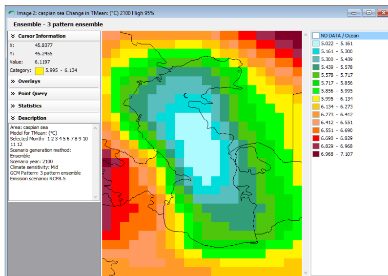
شکل ۵: پیش بینی ضریب تغییرات دمای حوضه دریای خزر (۱۹۸۱-۲۱۰۰) RCP 8.5
