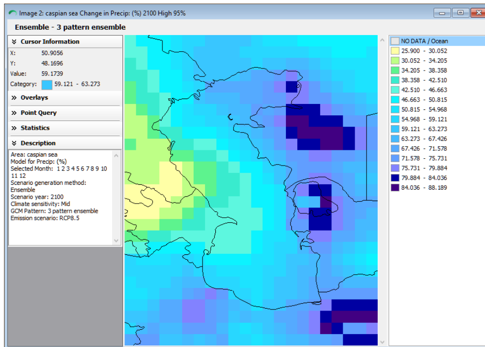
شکل ۳- پیش بینی ضریب تغییرات بارش حوضه دریای خزر (۲۱۰۰-۱۹۸۱) RCP 8.5
