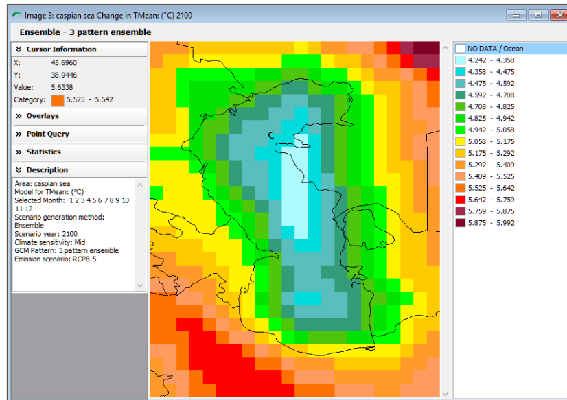
شکل ۴: پیش بینی توزیع مکانی درصد تغییرات دمای نسبت به میانگین پایه (۱۹۸۱-۲۱۰۰) RCP8.5
