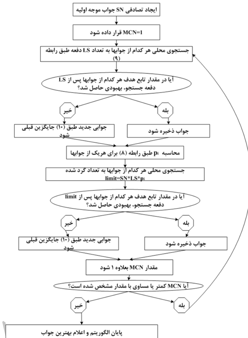
شکل ۳. فلوچارت نحوه عملکرد الگوریتم ABC ارائه شده
