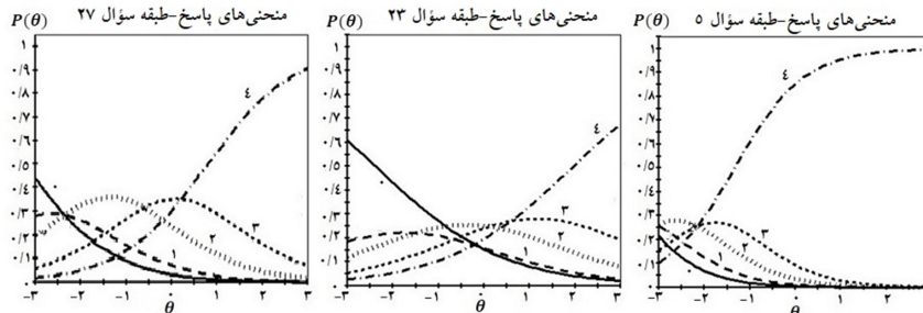
شکل ۳. منحنی‌های پاسخ-طبقه سؤال‌های ۵، ۲۳ و ۲۷ مقیاس سنجش توانایی‌های شناختی در مدل تک بُعدی
