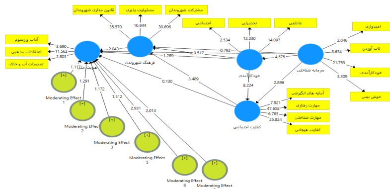
شکل ۲. نتایج آزمون Bootstrapp برای تعیین آماره t ضریب مسیر
