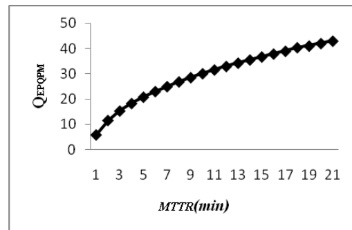
شکل ۳. نمودار رفتار QEPQPM بر اساس تغییرات MTTR
