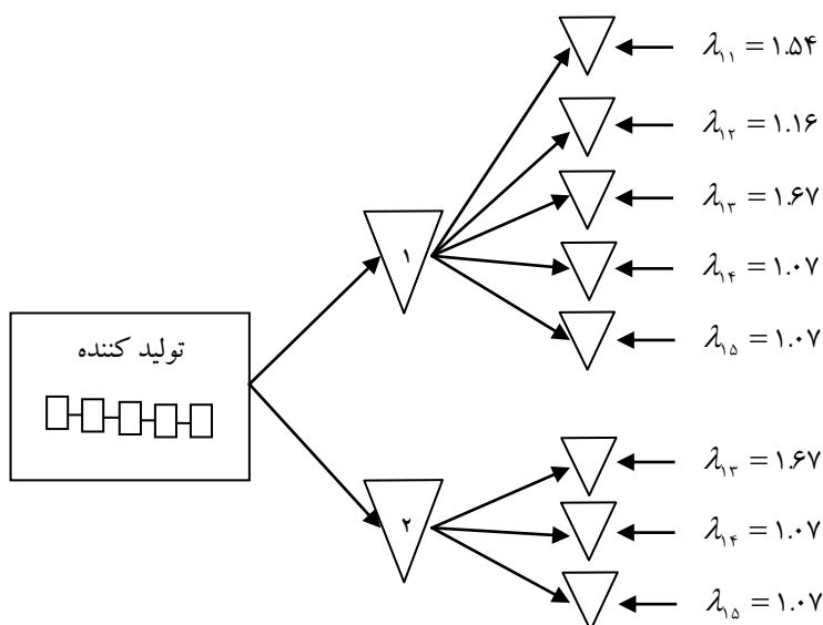
شکل ۱. سیستم موجودی سه سطحی و چند لایه مورد بررسی
