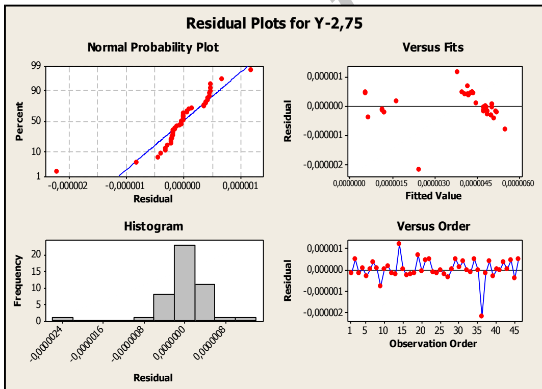
شکل ۳. نمودارهای مانده‌ها برای متغیر پاسخ تبدیل یافته y^{-۲.۷۵}
