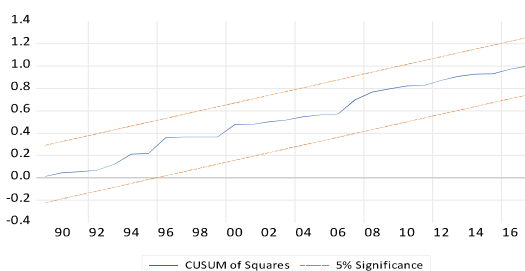
آزمون CUSUMq
