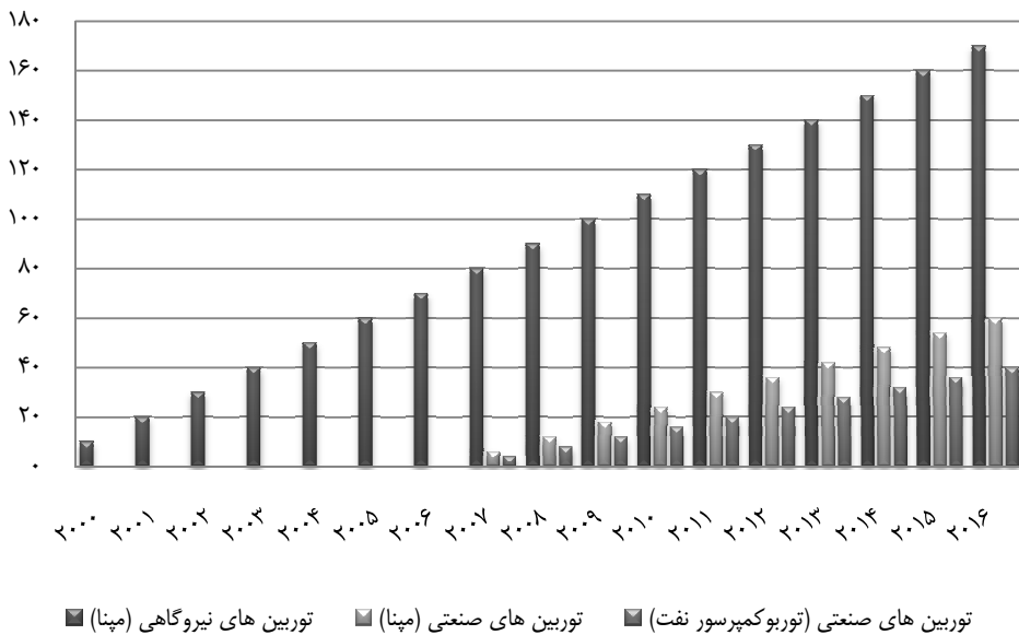
شکل ۱) تولید انباشتی توربین‌های گازی نیروگاهی و صنعتی توسط شرکت‌های توگا و OTC
