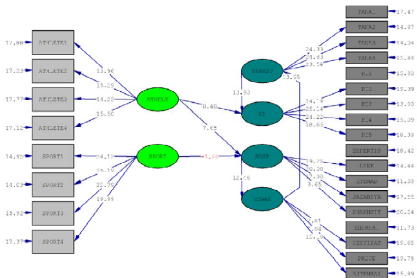
شکل ۱. نتایج مدل‌سازی معادلات ساختاری متغیرهای پژوهش بر اساس بار عاملی استاندارد شده
