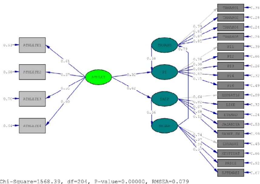
شکل ۳. مدل اصلاح شده بر اساس ضرایب استاندارد
