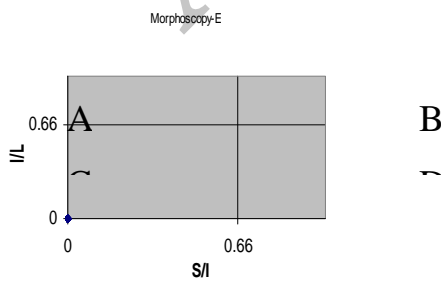
نمودار 25-2- تغییرات مورفوسکوپی ذرات رسوبی
