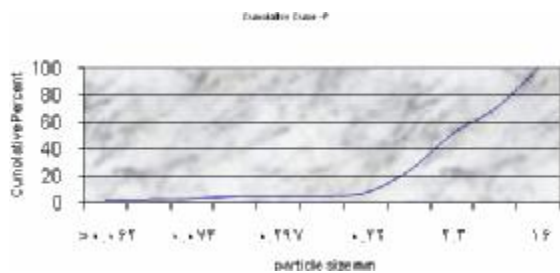
نمودار 2-8- نمودار تجمعی
