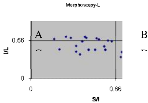
نمودار 23-2- تغییرات مورفوسکوپی ذرات رسوبی
