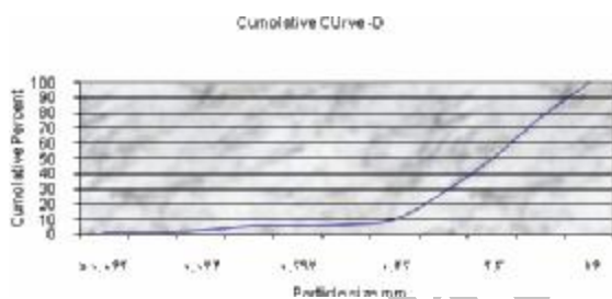
نمودار 2-10- نمودار تجمعی
