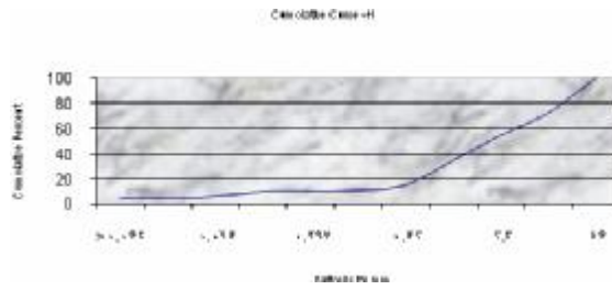
نمودار 21-2- نمودار تجمعی
