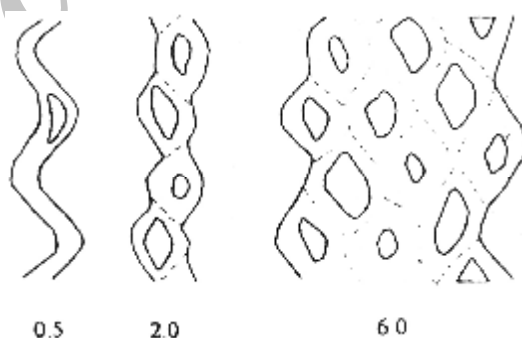
شکل 1-7- پارامتر سدی کانال منفرد 0/5، مولتی کانالها با پارامتر سدی
