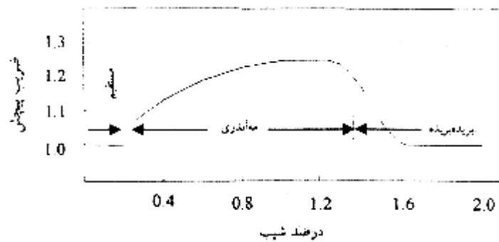
نمودار 2-7- ارتباط بین ضریب پیچش و درصد شیب (شام و خان 1972،
