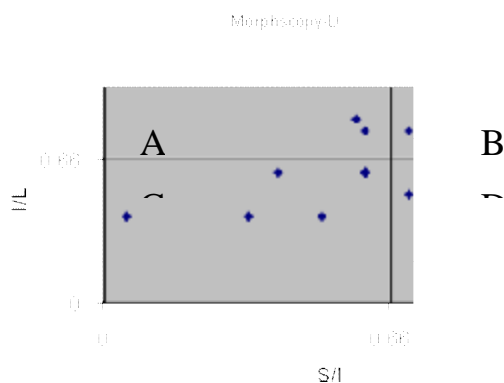
نمودار 2-28- تغییرات مورفوسکوپی ذرات رسوبی
