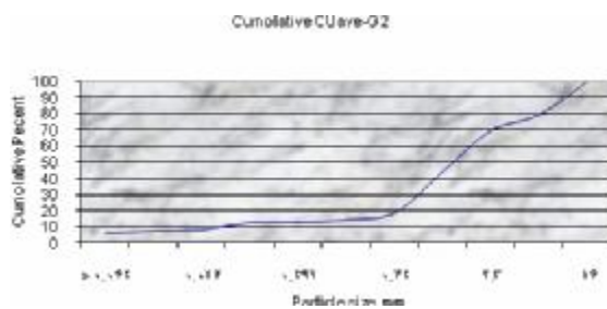
نمودار 2-5- نمودار تجمعی
