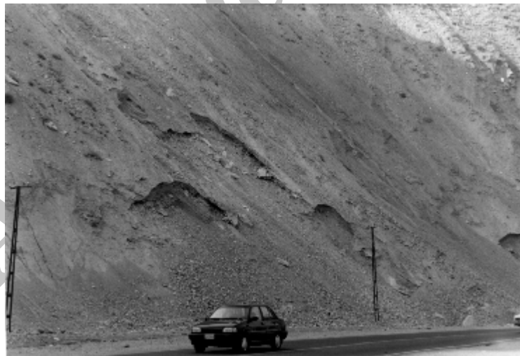
عکس 6-2- فرسایش ورقه‌ای نزدیک روستای گلوگان (دید به سمت غرب)
