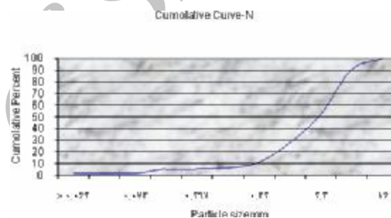
نمودار 2-1- نمودار تجمعی
