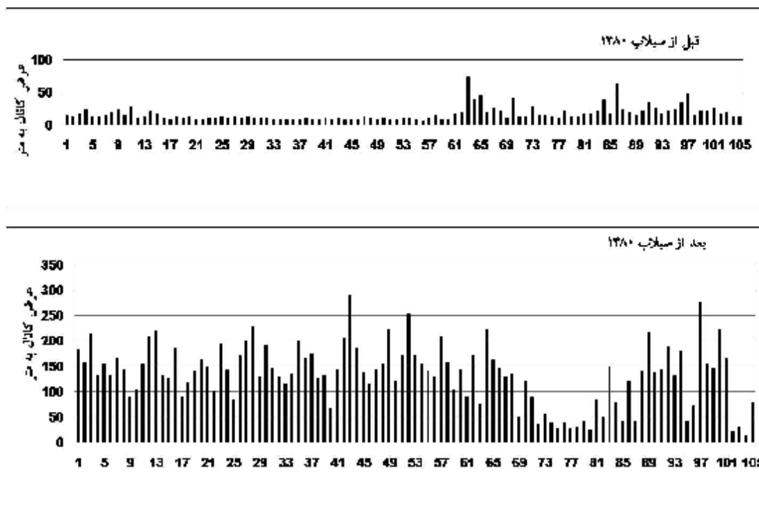
شکل شماره 7- تغییرات عرض کانال اصلی قبل و بعد از سیلاب 1380 در محل مقاطع نمونه
