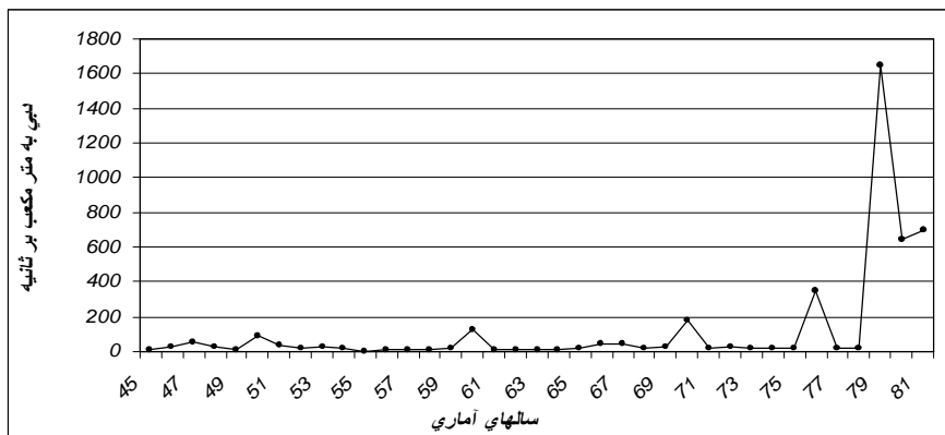
شکل شماره 3- نمودار مقادیر حداکثرهای دبی لحظه‌ای حوضه‌ی مادرسو در ایستگاه هیدرومتری تنگراه (بر اساس مقادیر اعلام شده توسط وزارت نیرو)
