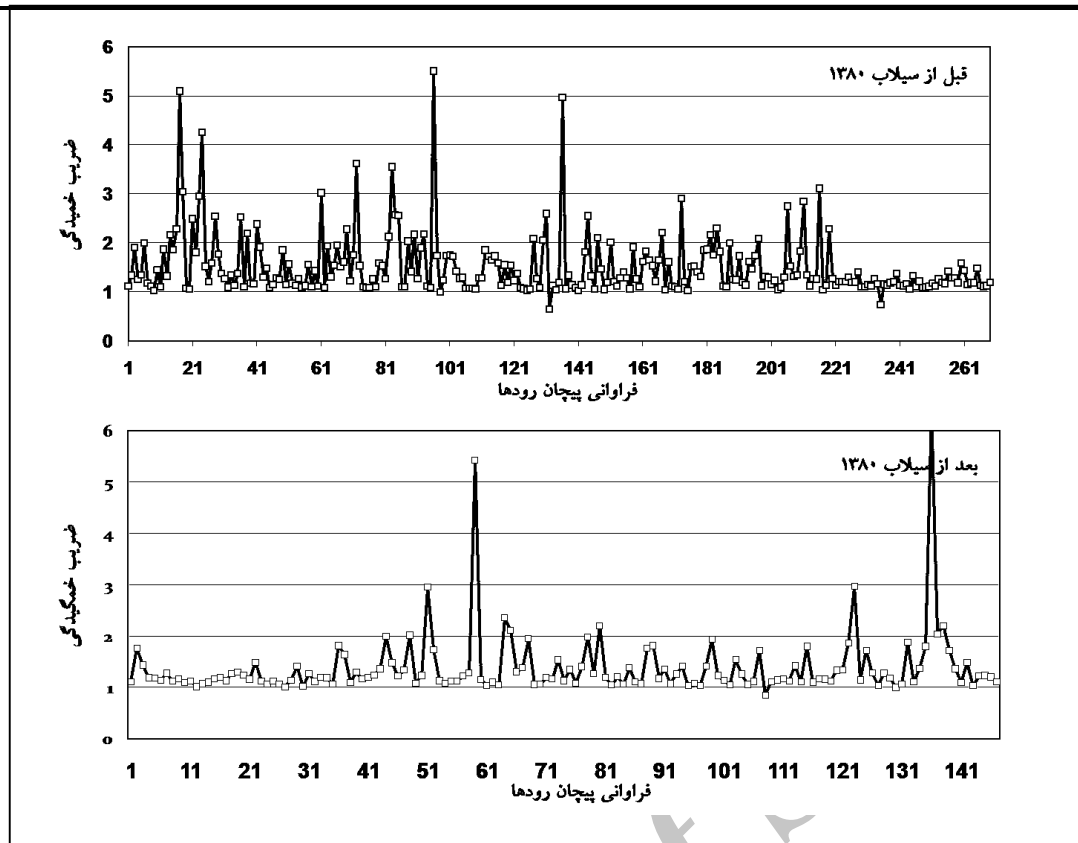
شکل شماره 8- تغییر فراوانی و ژئومتری مناندرها در بستر اصلی رود
