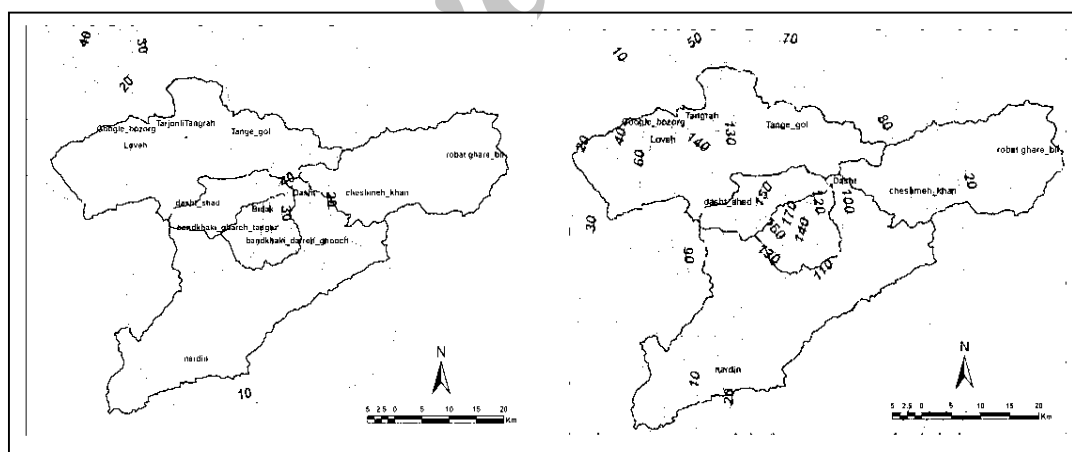
شکل شماره 2- وضعیت بارش در روزهای 19 و 20 مرداد 1380 ( جایکا، 2005، ص 63-2)
