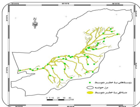
شکل ۵: نقاط روستاها در معرض خطر متوسط سیل در حوزه گرگانرود
