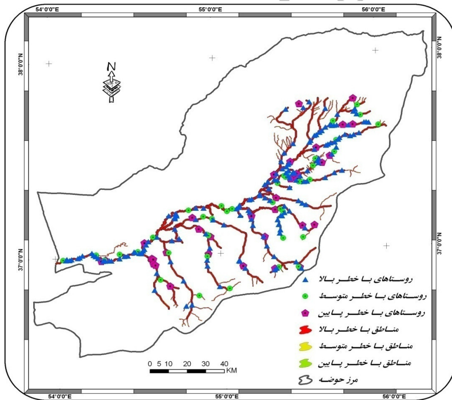
شکل ۷) پراکنش روستاهای در پهنه‌های مختلف خطر سیل خیزی
