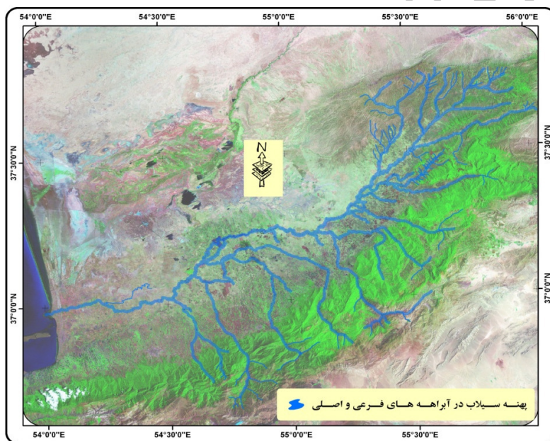
شکل ۸) پهنه‌های در معرض آب‌گرفتگی ناشی از سیلاب
